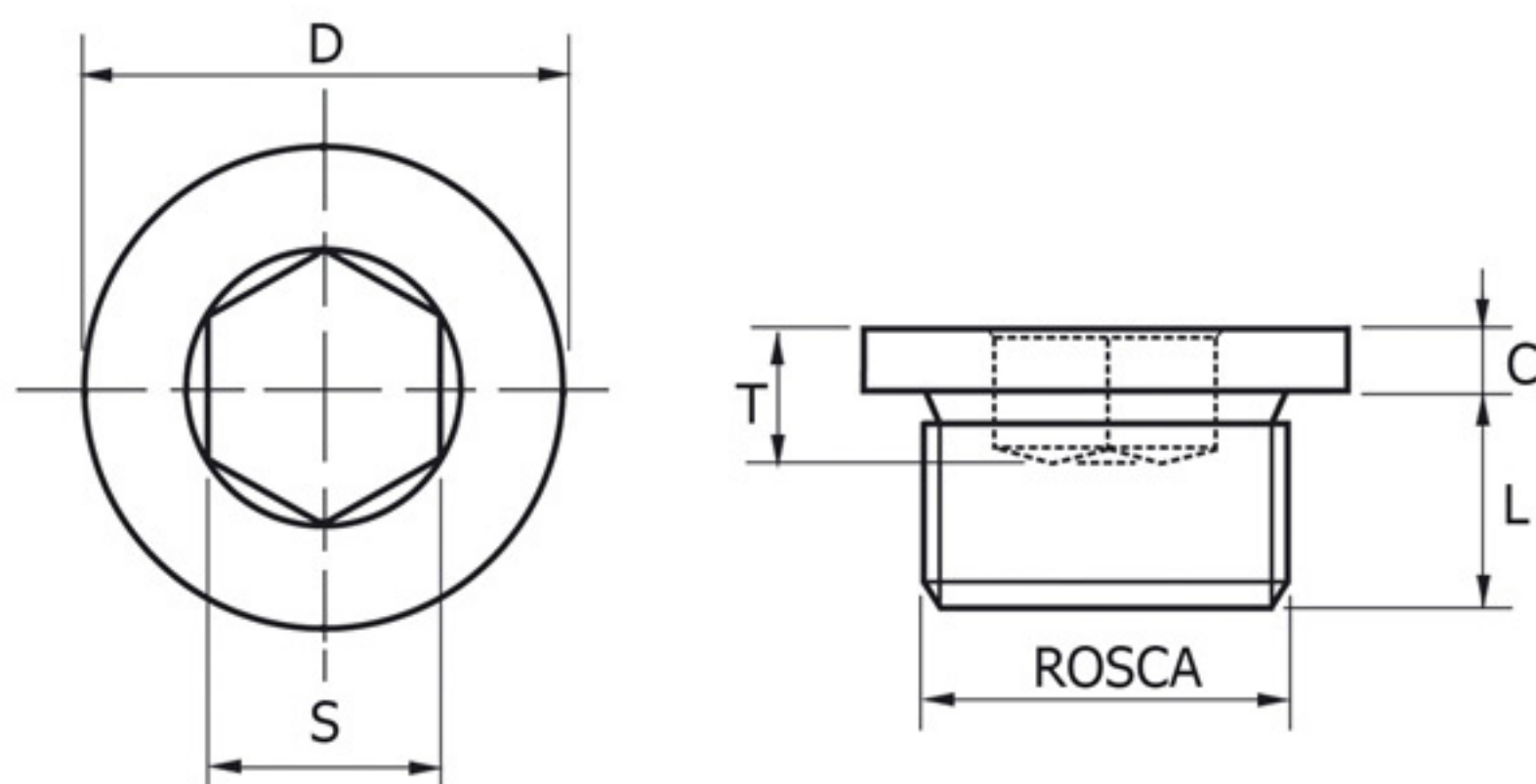
DIN 908 - Rosca BSP
